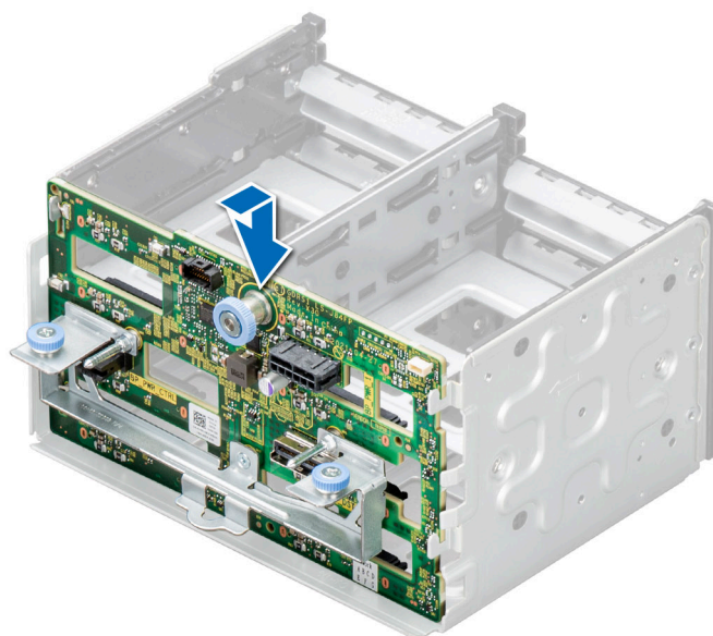
Ilustración 61. Instalación del backplane para unidades de 2,5 pulgadas
