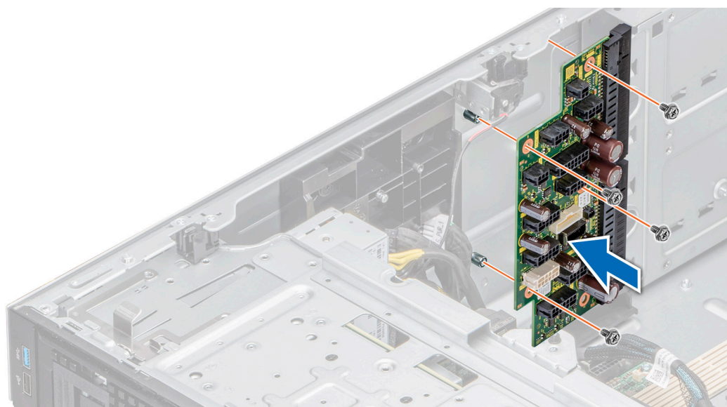
Ilustración 175. Instalación de la placa mediadora de alimentación
