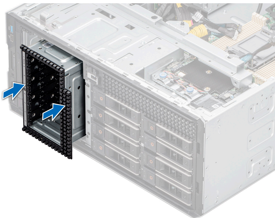
Ilustración 71. Instalación de una bahía de unidad de NVMe
