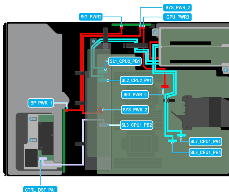
Ilustración 87. Enrutamiento de cables: 8 SAS de 3,5 pulgadas con dos soportes verticales para la GPU
