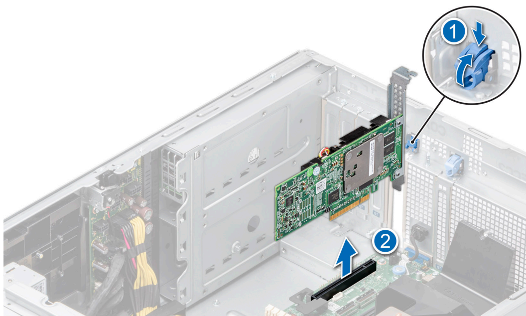
Ilustración 128. Extracción de una tarjeta de expansión
