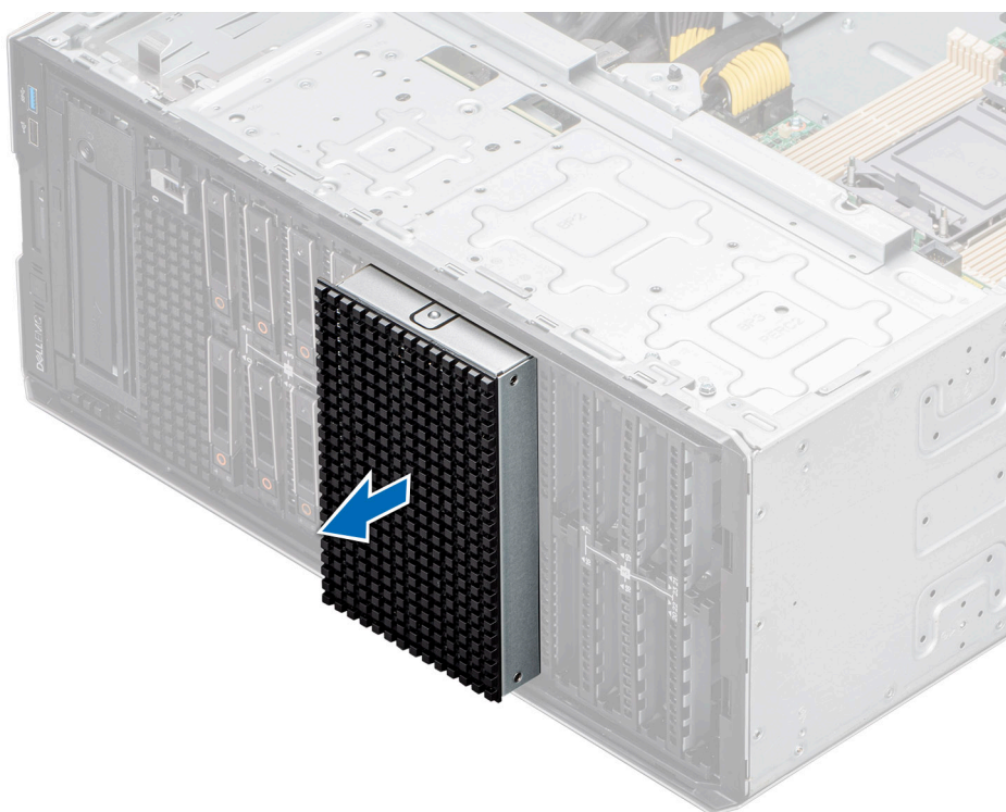
Ilustración 62. Extracción de la canastilla de relleno de la bahía de unidad
