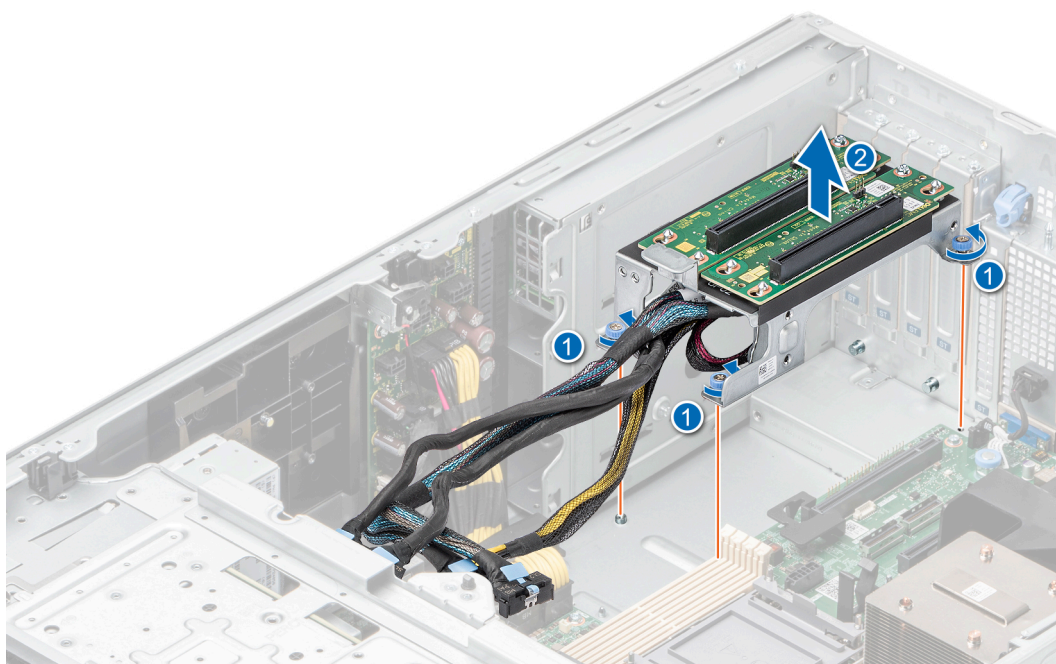
Ilustración 138. Extracción del soporte vertical de la GPU
