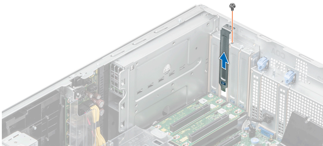
Ilustración 136. Extracción del soporte de relleno
