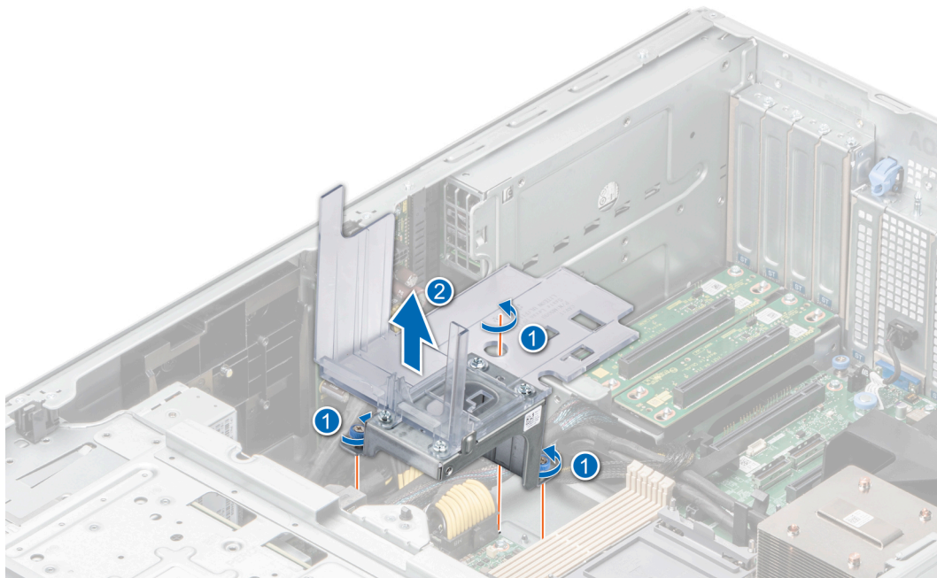
Ilustración 132. Extracción del soporte para tarjetas de la GPU
