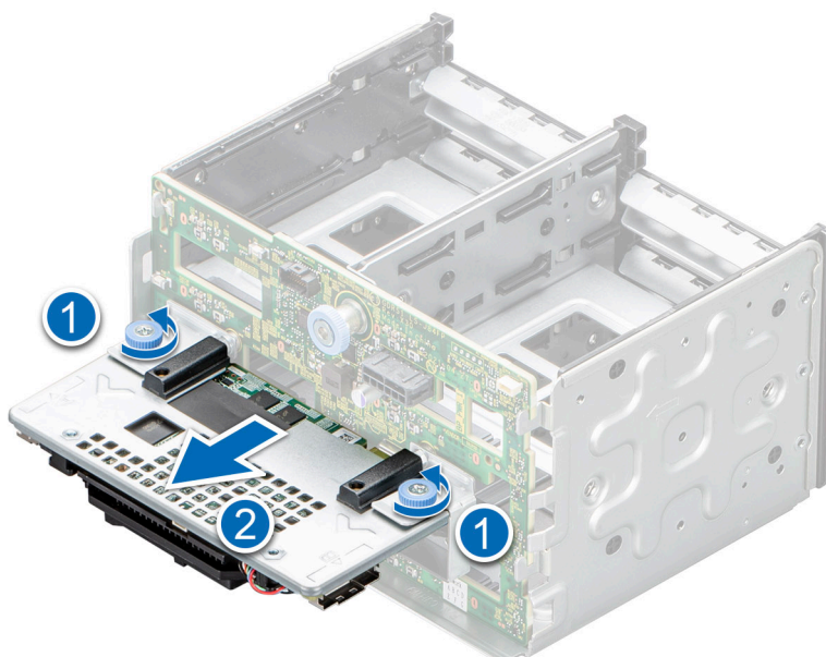
Ilustración 43. Extracción del módulo de PERC frontal en backplanes para unidades de 2,5 pulgadas.
