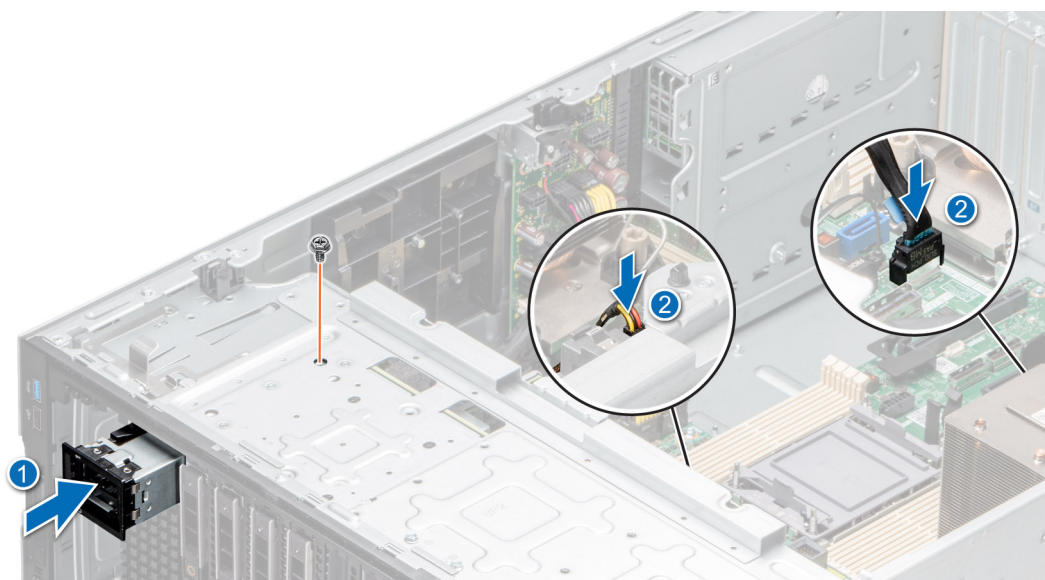
Ilustración 112. Instalación del módulo S2 de BOSS
