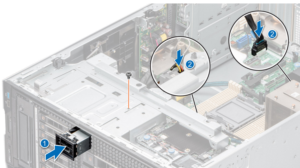
Ilustración 113. Instalación del módulo S2 de BOSS
