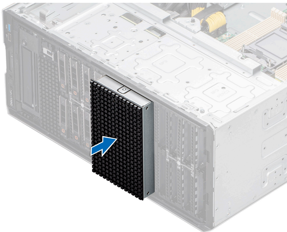
Ilustración 64. Instalación de la canastilla de relleno de la bahía de unidad
