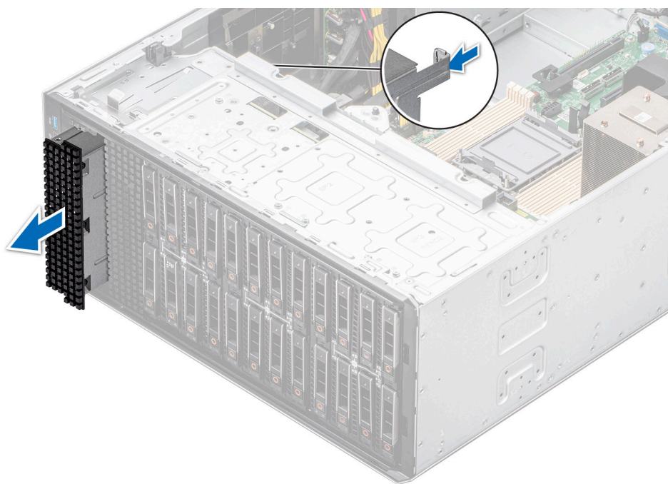
Ilustración 97. Extracción de la unidad de respaldo en cinta de relleno
