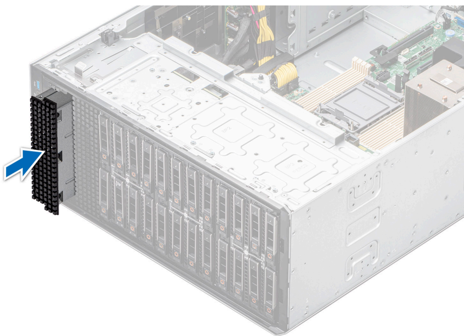
Ilustración 98. Instalación de la unidad de respaldo en cinta de relleno
