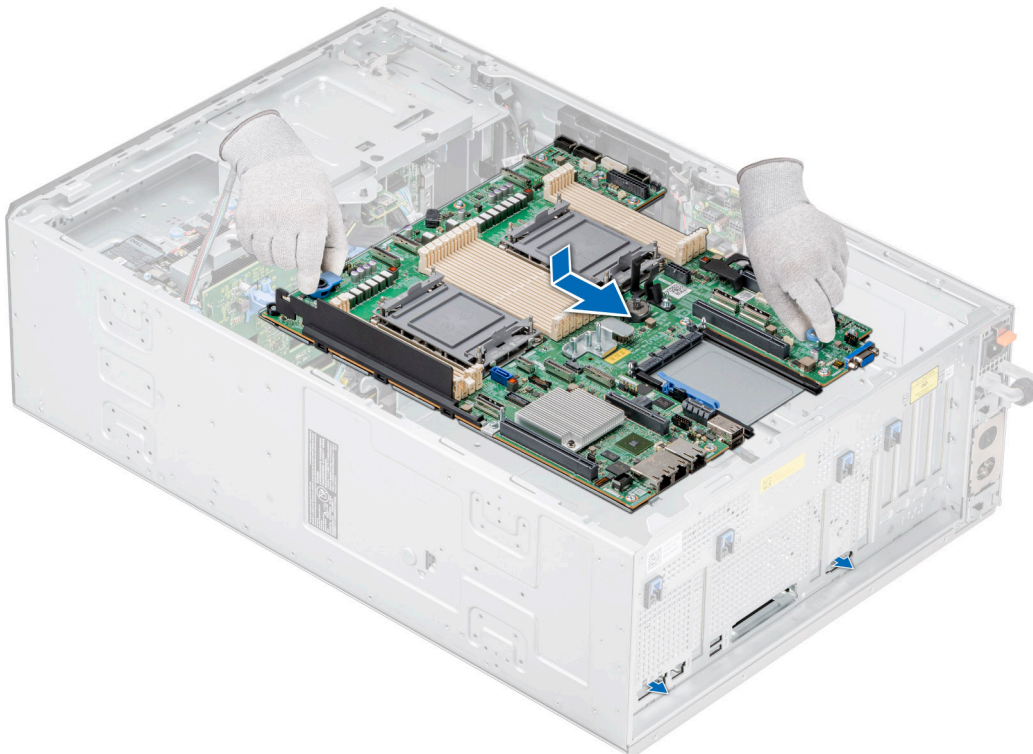
Ilustración 177. Instalación de la tarjeta madre
