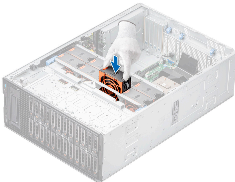
Ilustración 36. Instalación de un ventilador de refrigeración
