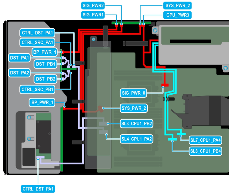
Ilustración 91. Enrutamiento de cables: 8 NVMe de 3,5 pulgadas + 8 de 2,5 pulgadas con el soporte vertical para la GPU
