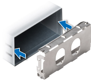
Ilustración 166. Instalación de una fuente de alimentación de relleno de 86 mm
