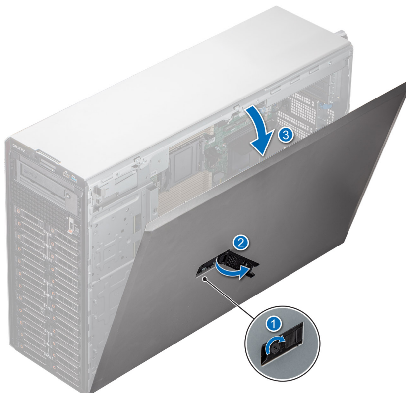
Ilustración 31. Extracción de la cubierta del sistema
