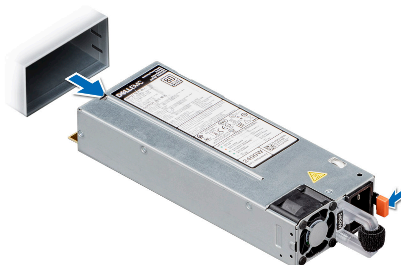
Ilustración 170. Extracción de una fuente de alimentación de 86 mm
