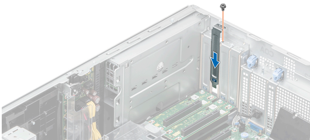
Ilustración 135. Instalación del soporte de relleno
