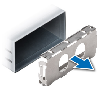
Ilustración 164. Extracción de una fuente de alimentación de relleno de 86 mm
