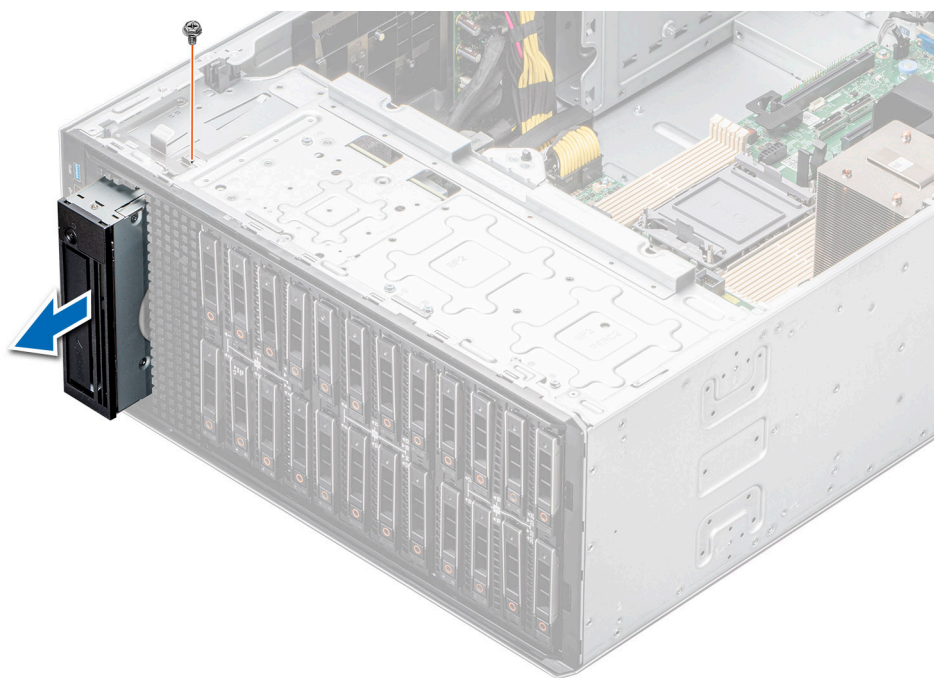
Ilustración 99. Extracción de la unidad de respaldo en cinta
