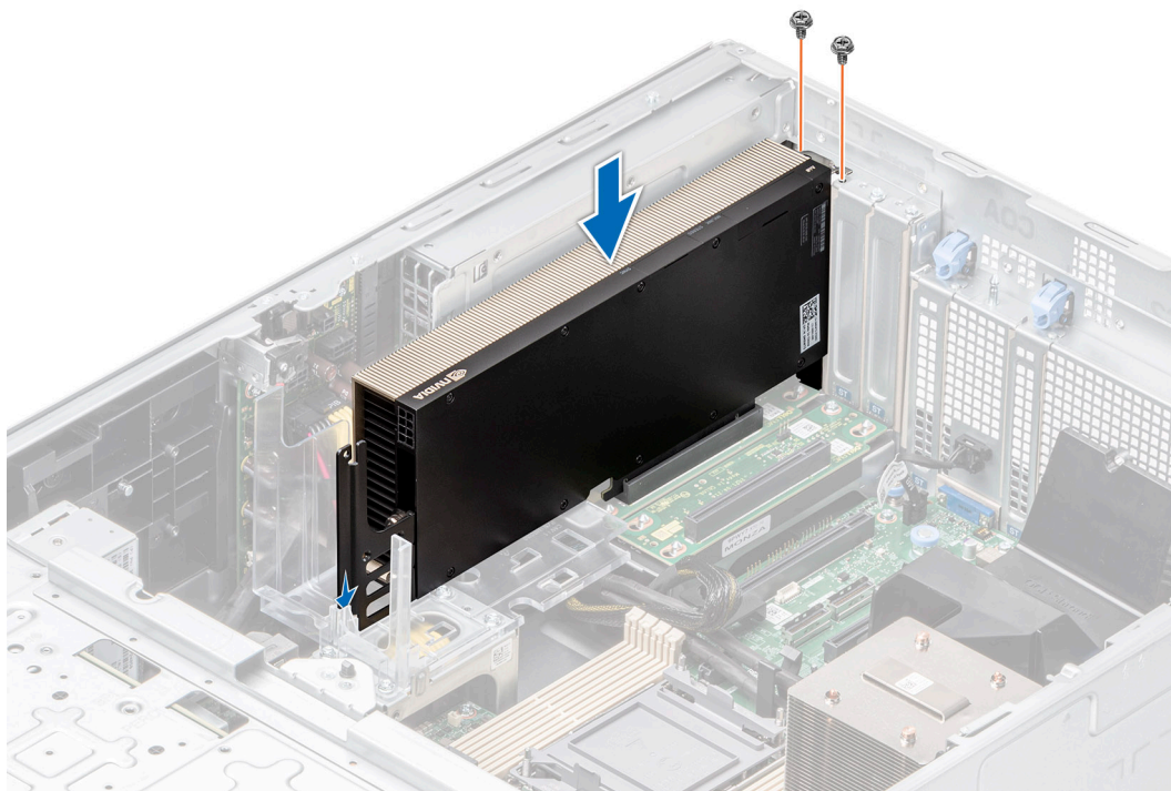
Ilustración 137. Instalación de la tarjeta GPU
