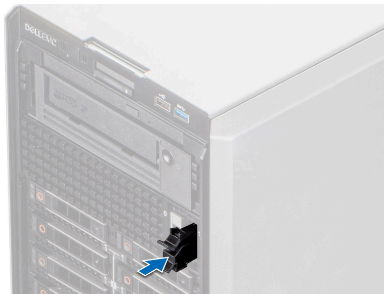
Ilustración 115. Instalación del soporte de tarjetas de relleno de Boot Optimized Storage Subsystem S2
