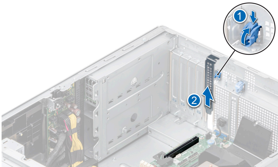
Ilustración 130. Extracción del soporte de relleno
