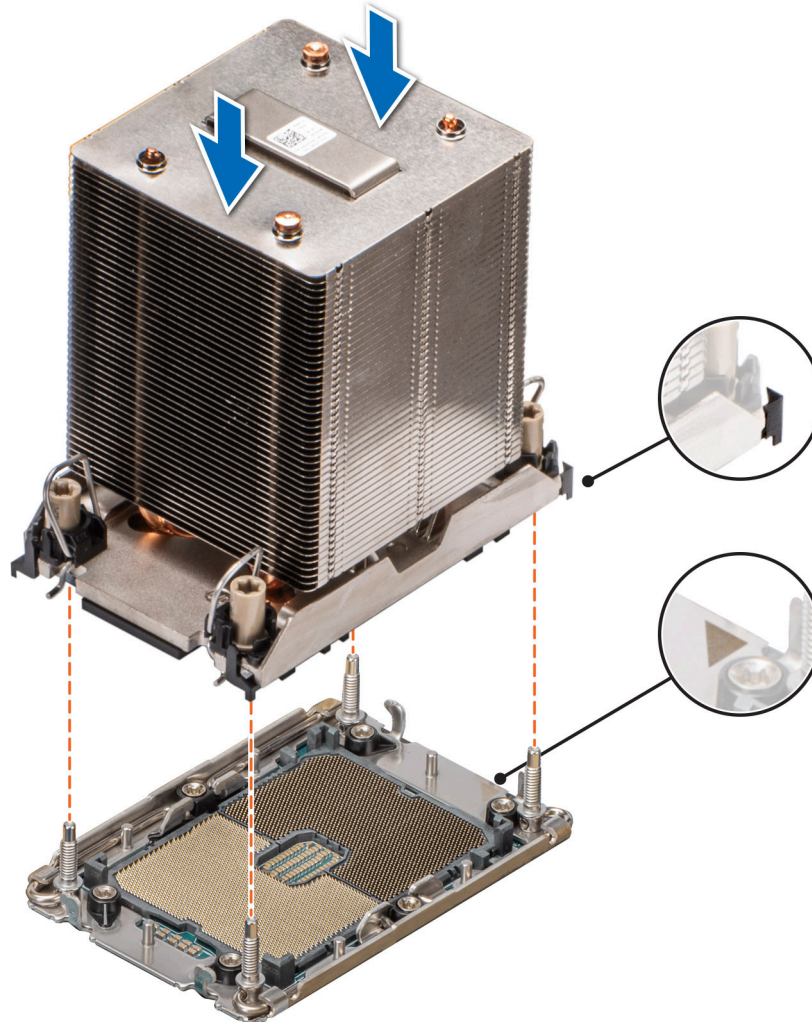
Ilustración 149. Instalación del disipador de calor del procesador
