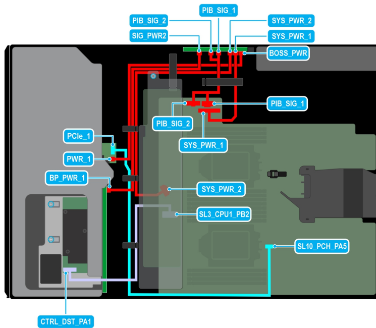
Ilustración 85. Enrutamiento de cables: 8 SAS de 3,5 pulgadas con el módulo BOSS S2
