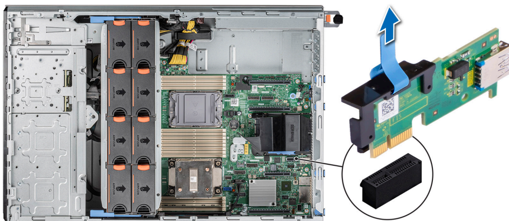
Ilustración 120. Extracción del módulo USB interno
