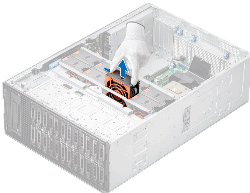
Ilustración 35. Extracción de un ventilador de refrigeración
