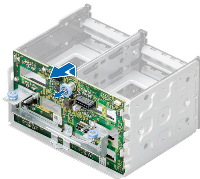
Ilustración 60. Extracción del backplane para unidades de 2,5 pulgadas
