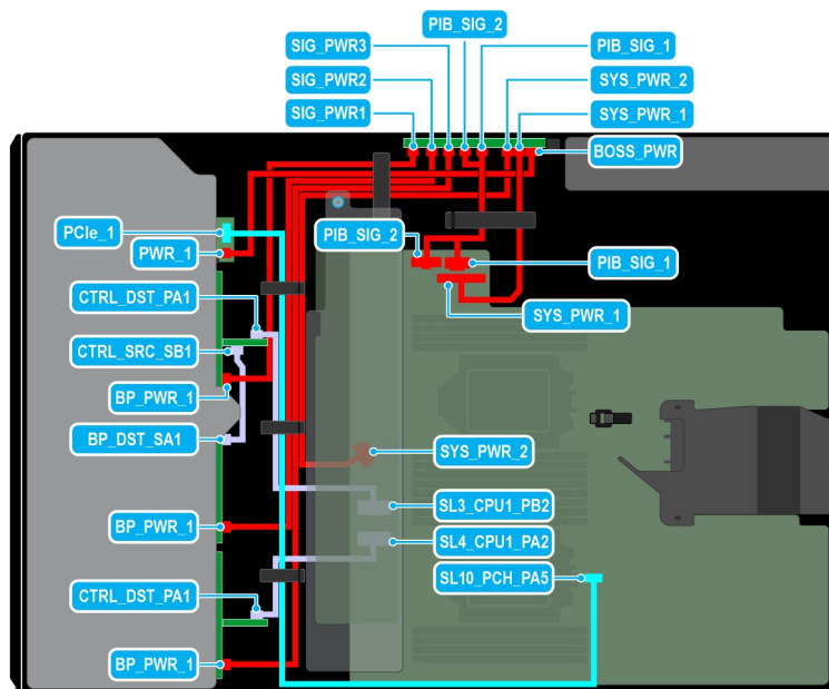
Ilustración 81. Enrutamiento de cables: 24 SAS de 2,5 pulgadas con el módulo BOSS S2
