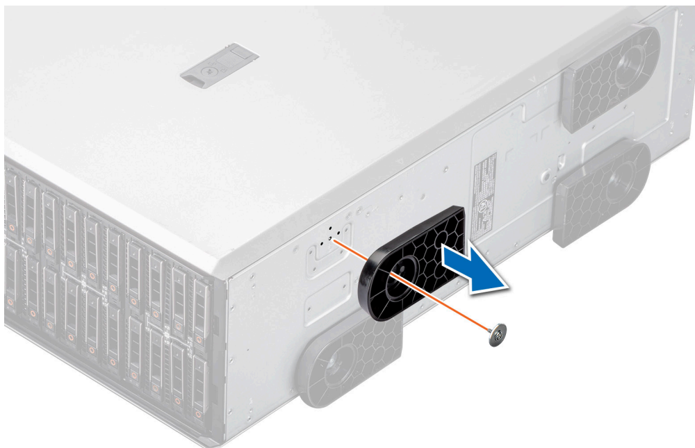
Ilustración 27. Extracción de los pies del sistema
