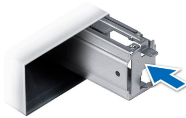
Ilustración 168. Instalación de un adaptador de fuente de alimentación
