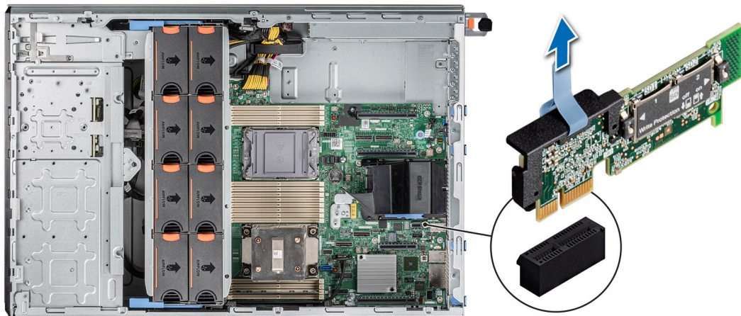
Ilustración 124. Extracción del módulo IDSDM
