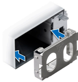
Ilustración 165. Instalación de una fuente de alimentación de relleno de 60 mm
