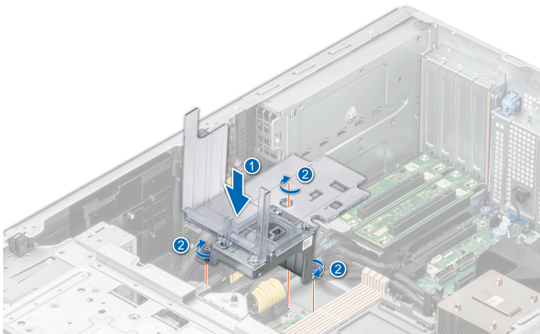
Ilustración 133. Instalación del soporte para tarjetas GPU
