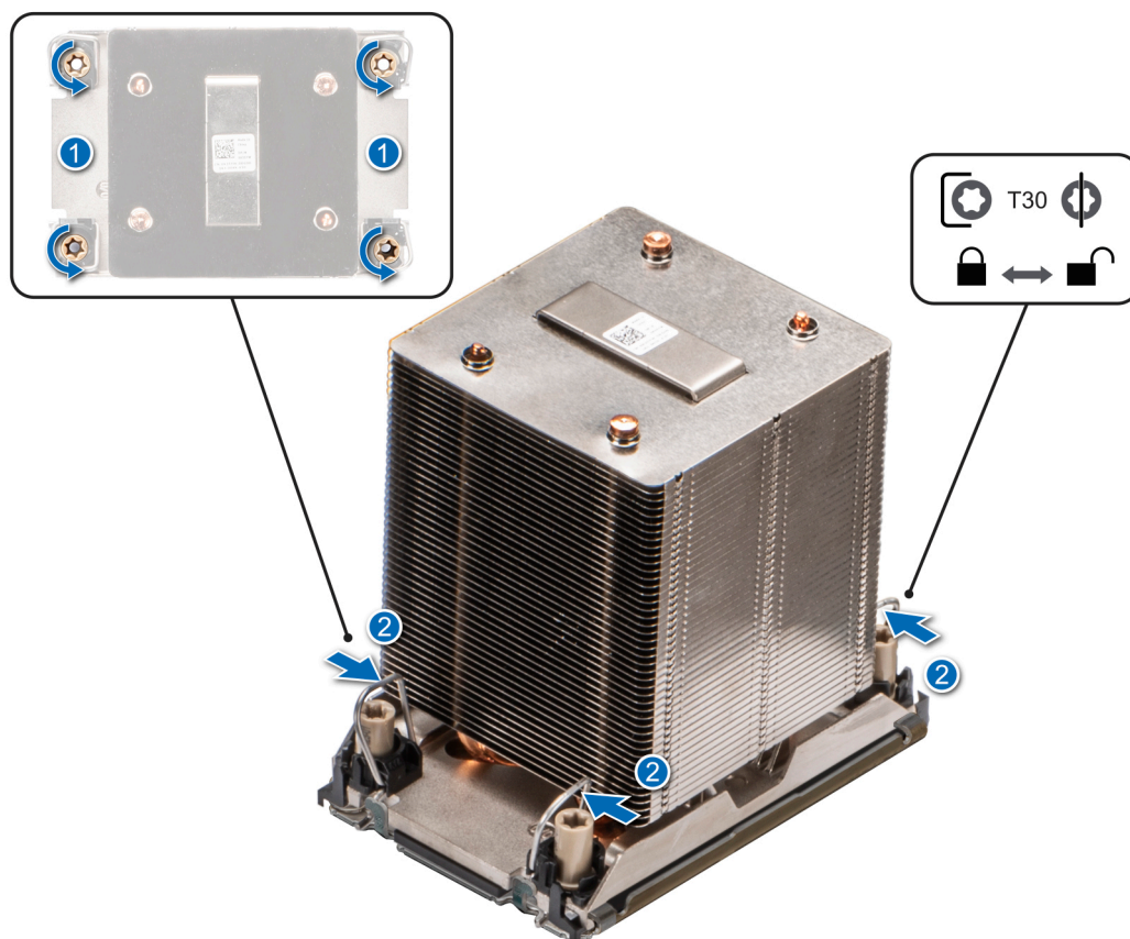
Ilustración 140. Extracción del módulo de disipador de calor del procesador.
