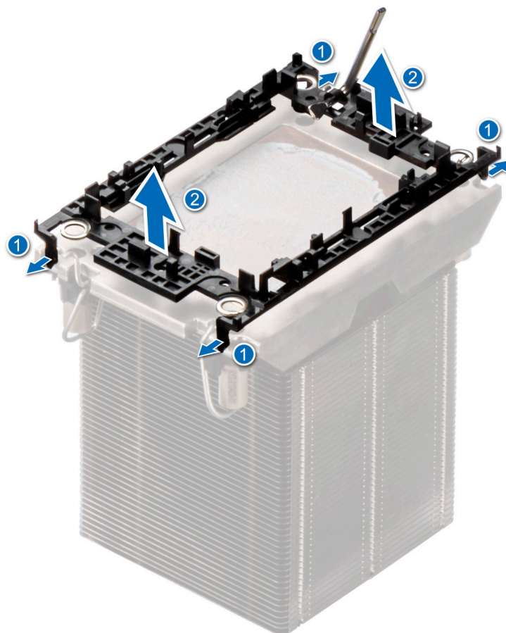
Ilustración 143. Extracción del gancho de retención
