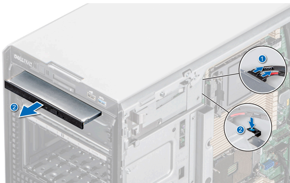
Ilustración 95. Extracción de la unidad óptica
