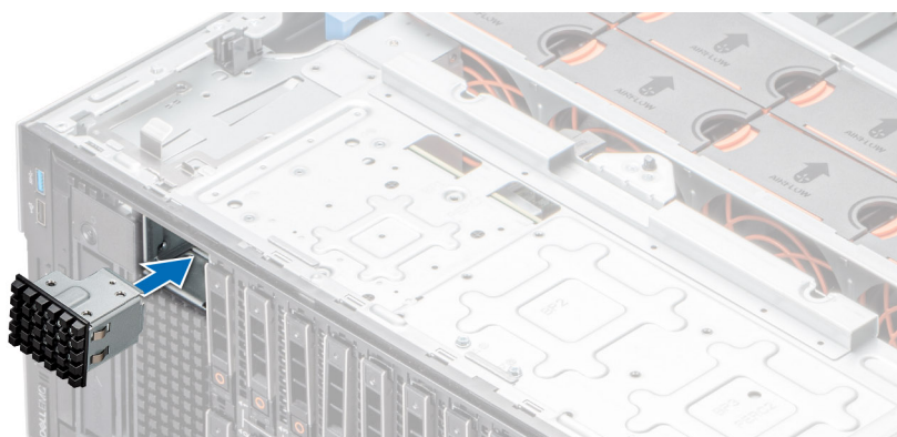
Ilustración 110. Instalación del módulo de Boot Optimized Storage Subsystem S2 de relleno
