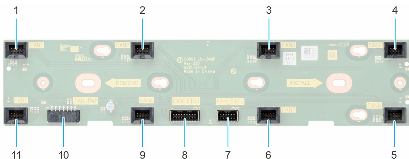
Ilustración 39. Conectores de la placa del ventilador
