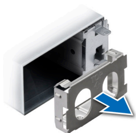
Ilustración 163. Extracción de una fuente de alimentación de relleno de 60 mm
