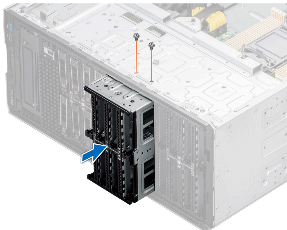
Ilustración 69. Instalación de una bahía de unidad
