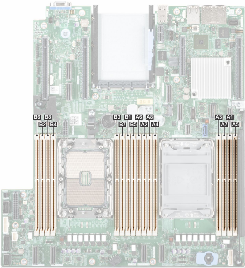
Ilustración 105. Canales de la memoria
