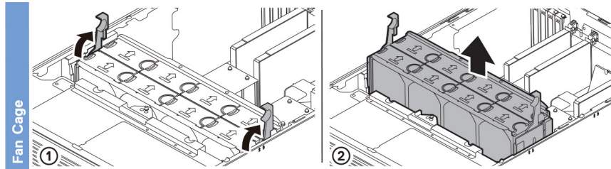
Ilustración 20. Canastilla del ventilador
