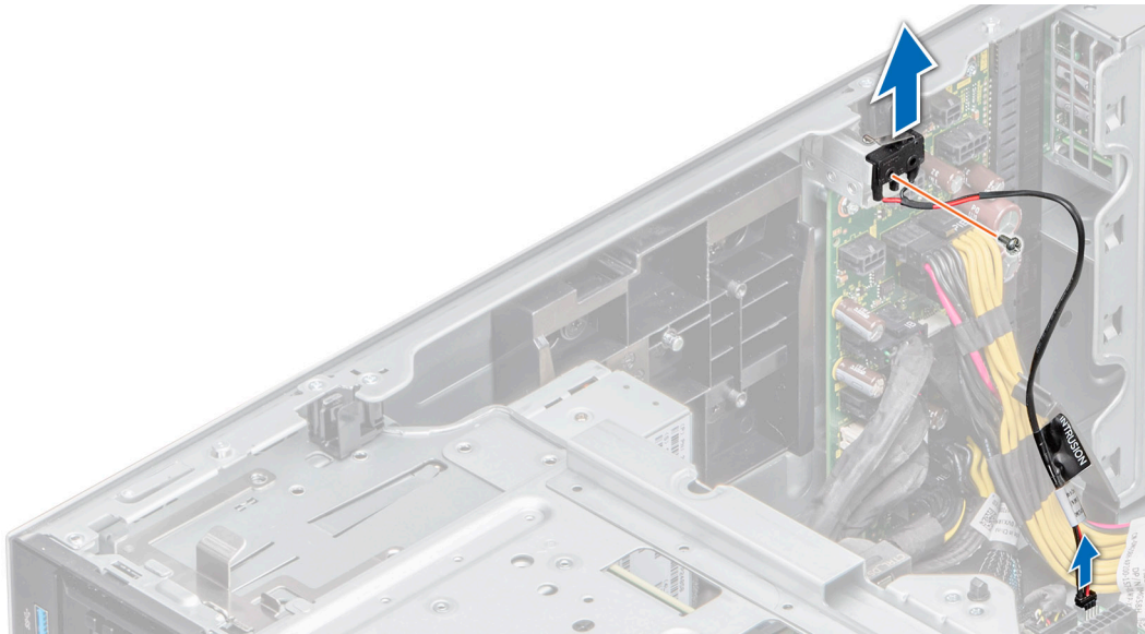
Ilustración 161. Extracción del módulo del interruptor de intrusiones
