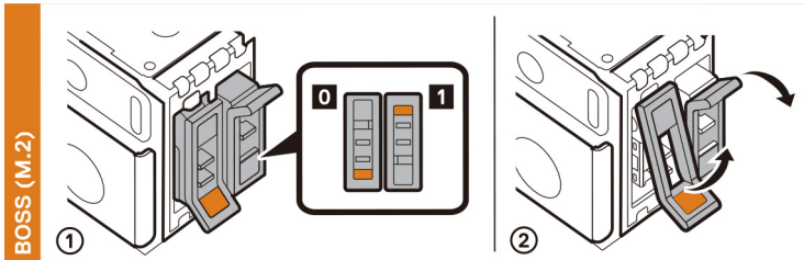
Ilustración 14. Módulo de Boot Optimized Storage Subsystem S2
