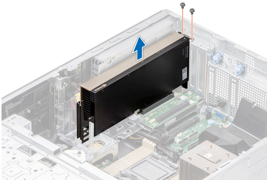
Ilustración 134. Extracción de la tarjeta GPU
