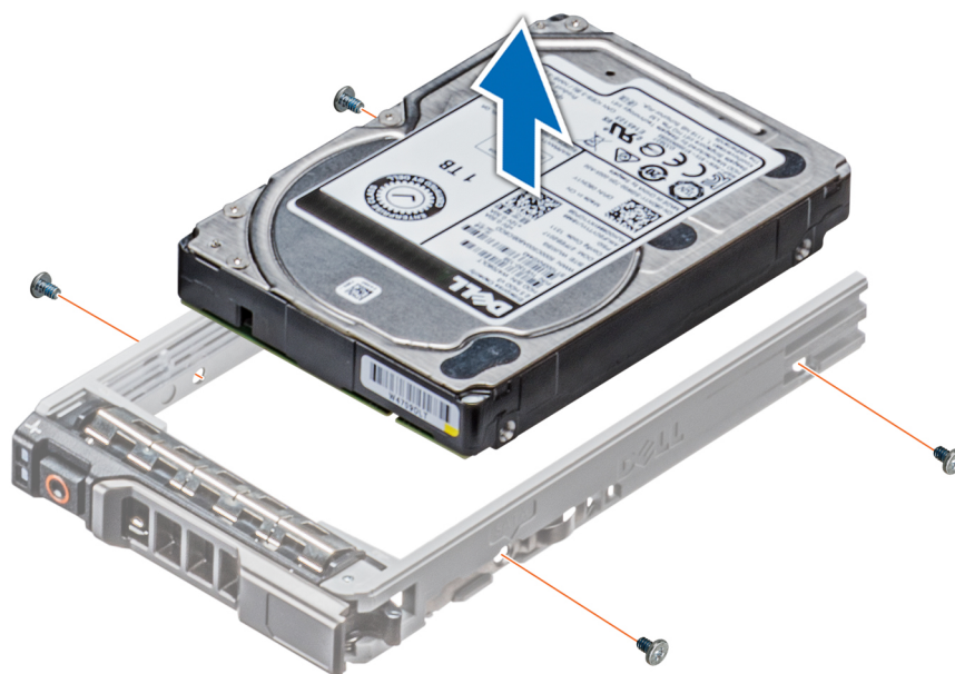
Ilustración 50. Extracción de una unidad del portaunidades
