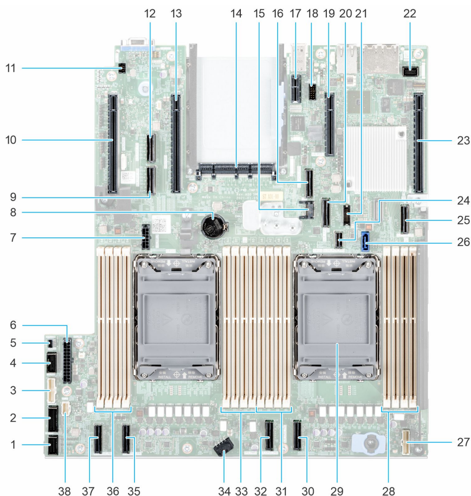
Ilustración 179. Puentes y conectores de la tarjeta madre del sistema
