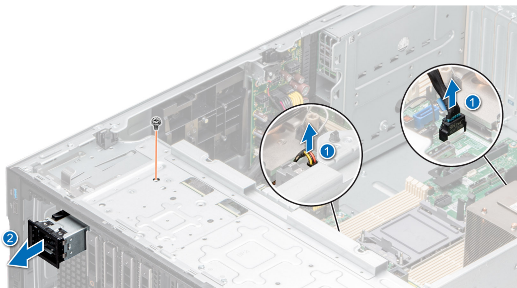
Ilustración 108. Extracción del módulo S2 de BOSS
