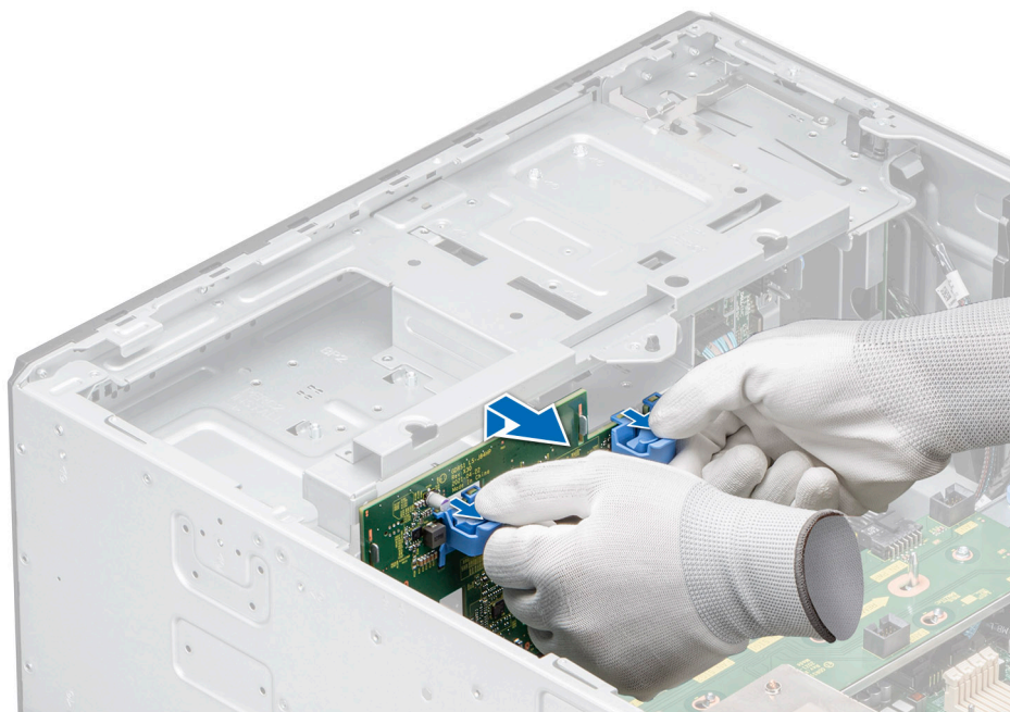
Ilustración 58. Extracción del backplane para unidades de 3,5 pulgadas
