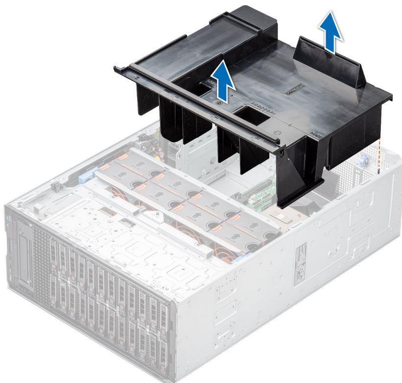
Ilustración 33. Extracción de la cubierta para flujo de aire
