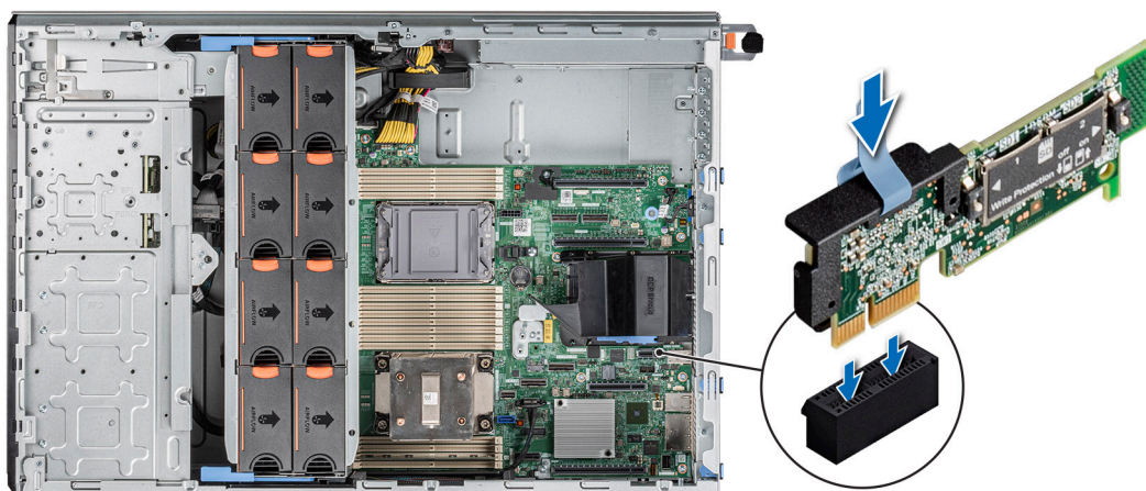
Ilustración 125. Instalación del módulo IDSMD
