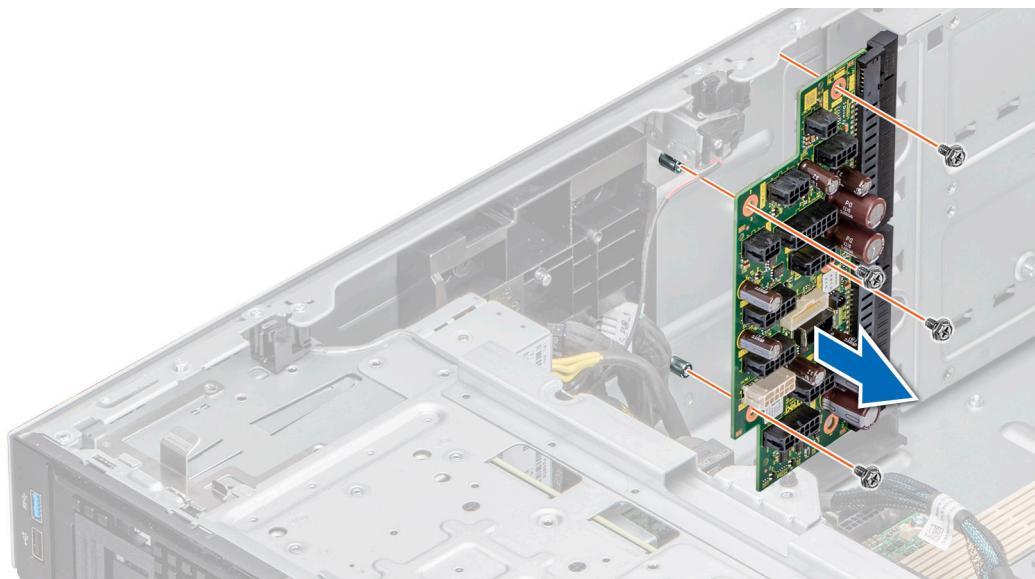
Ilustración 174. Extracción de la tarjeta PIB
