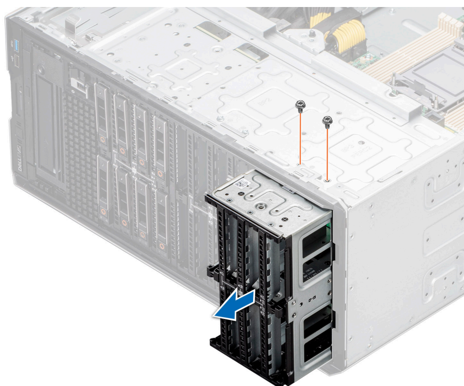
Ilustración 67. Extracción de una bahía de unidad
