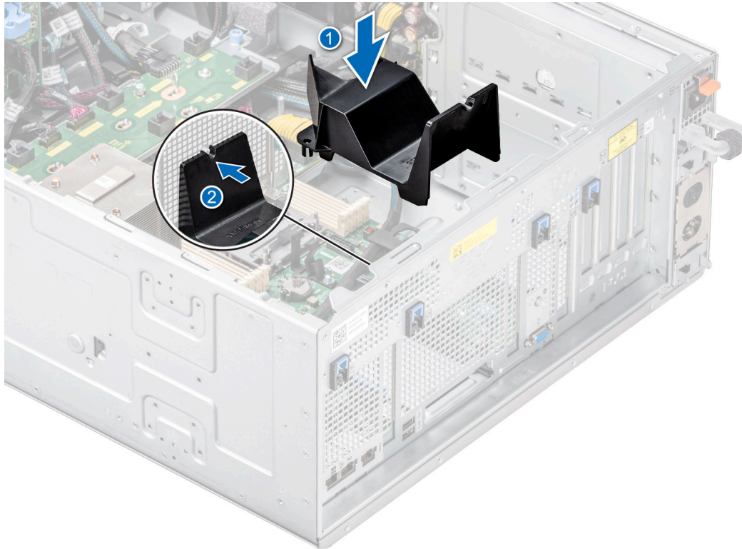
Ilustración 156. Instalación de la cubierta para flujo de aire de OCP.
