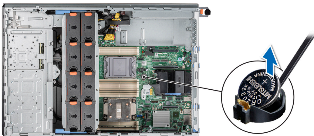
Ilustración 159. Extracción de la batería del sistema
