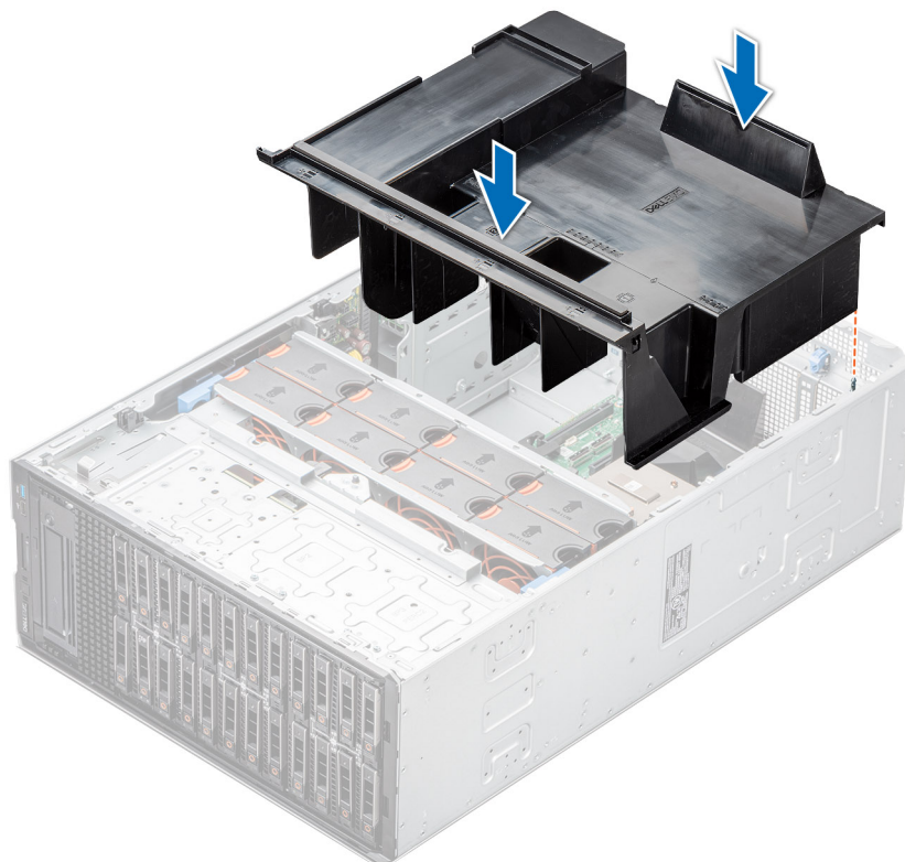
Ilustración 34. Instalación de la cubierta para flujo de aire
