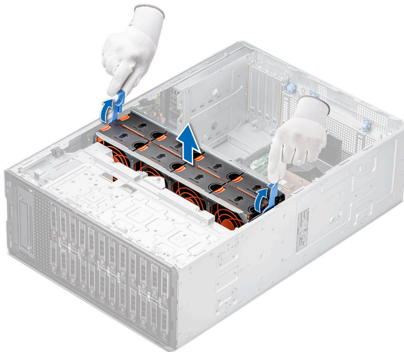
Ilustración 37. Extracción del compartimento del ventilador de refrigeración
