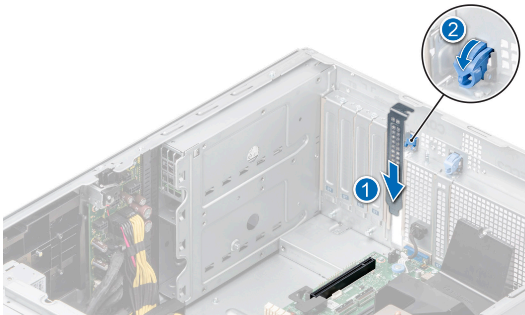
Ilustración 129. Instalación del soporte de relleno
