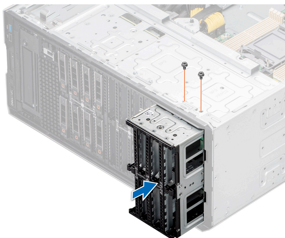
Ilustración 70. Instalación de una bahía de unidad
