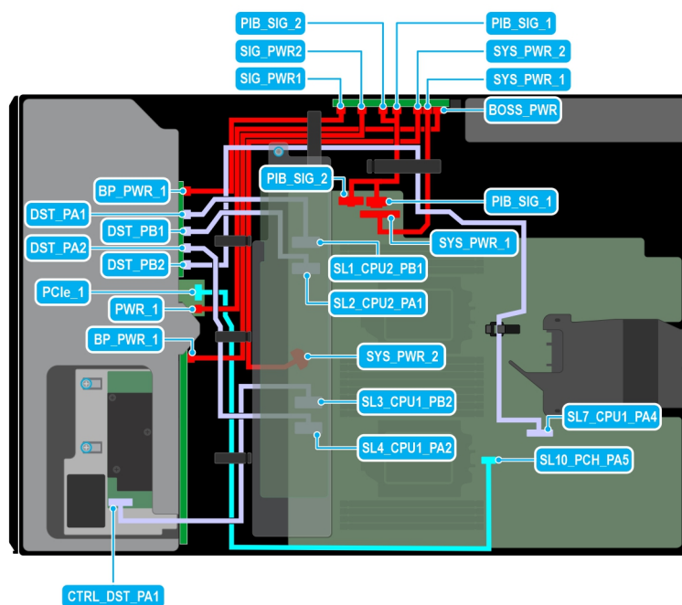
Ilustración 90. Enrutamiento de cables: 8 NVMe de 3,5 pulgadas + 8 de 2,5 pulgadas con el módulo BOSS S2
