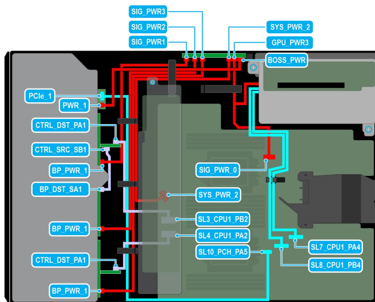
Ilustración 82. Enrutamiento de cables: 24 SAS de 2,5 pulgadas con soporte vertical para la GPU
