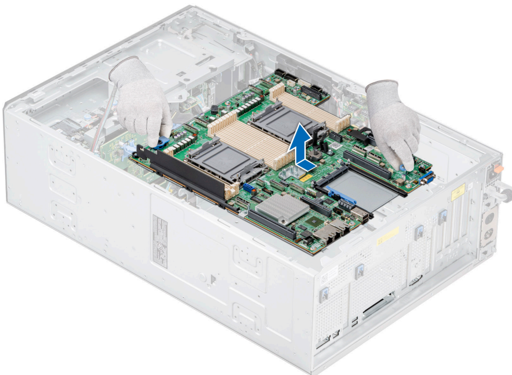
Ilustración 176. Extracción de la tarjeta madre
