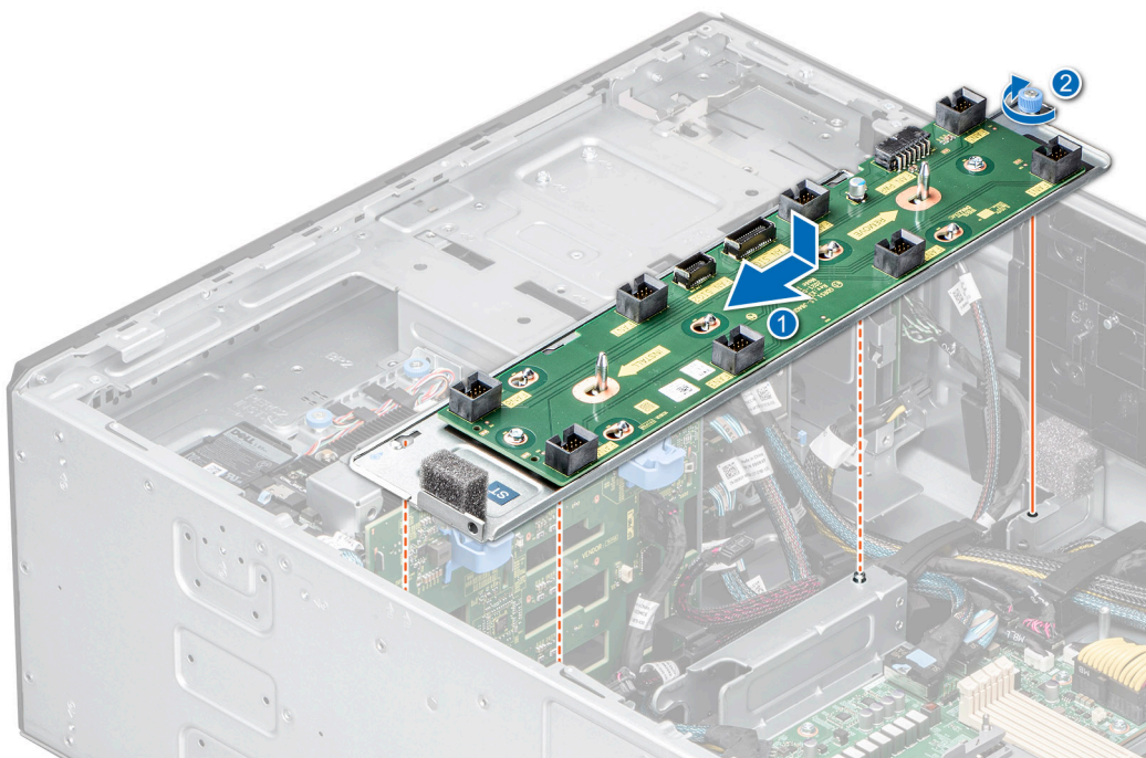
Ilustración 41. Instalación de la bandeja de la placa del ventilador
