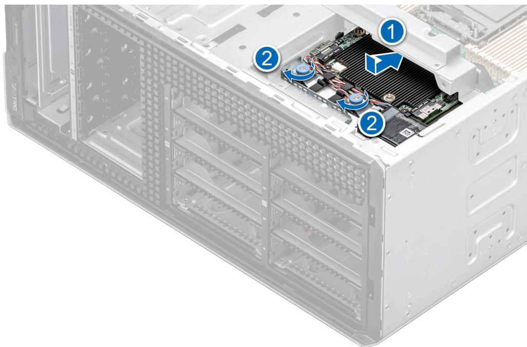
Ilustración 44. Instalación del módulo de PERC frontal en backplanes para unidades de 3,5 pulgadas.
