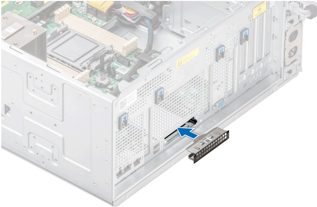
Ilustración 153. Instalación del soporte de relleno
