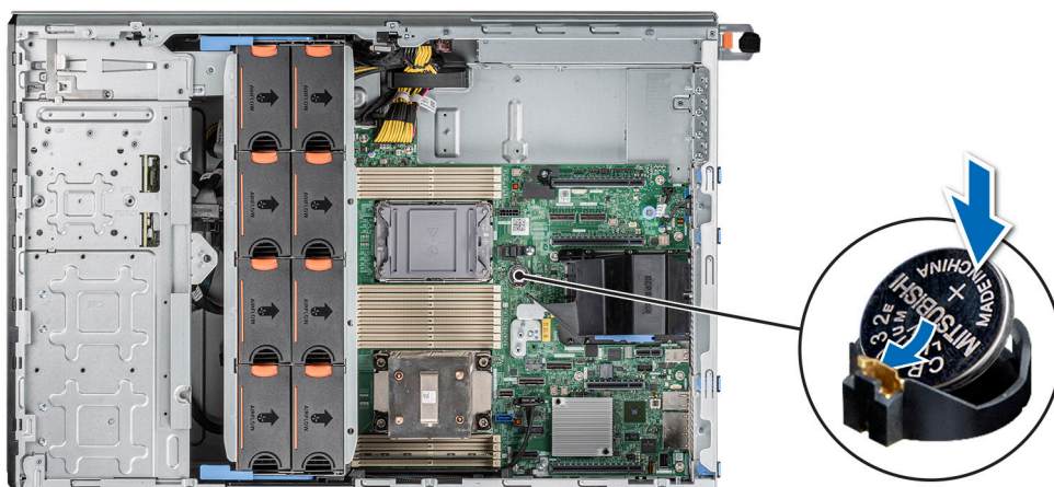
Ilustración 160. Instalación de la batería del sistema
