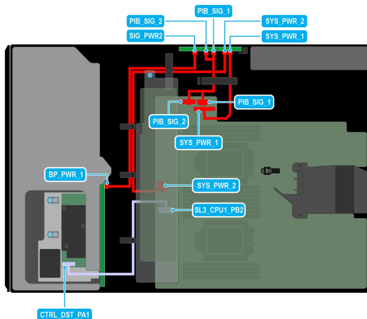
Ilustración 84. Enrutamiento de cables: 8 SAS de 3,5 pulgadas
