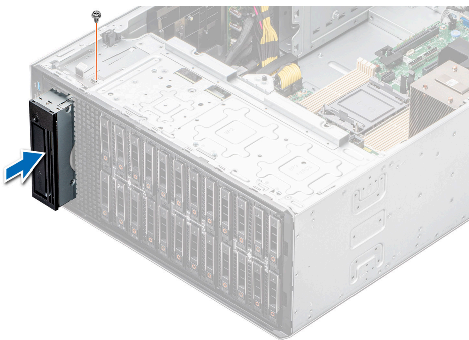
Ilustración 100. Instalación de la unidad de respaldo en cinta
