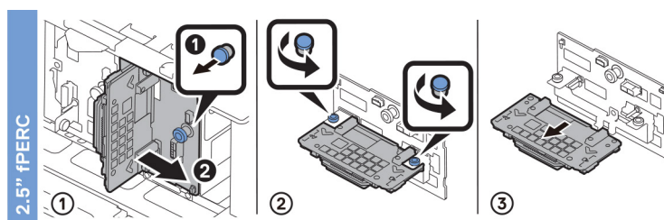
Ilustración 16. PERC frontal de 2,5 pulgadas
