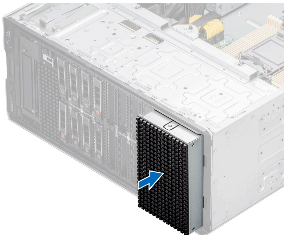
Ilustración 65. Instalación de la canastilla de relleno de la bahía de unidad
