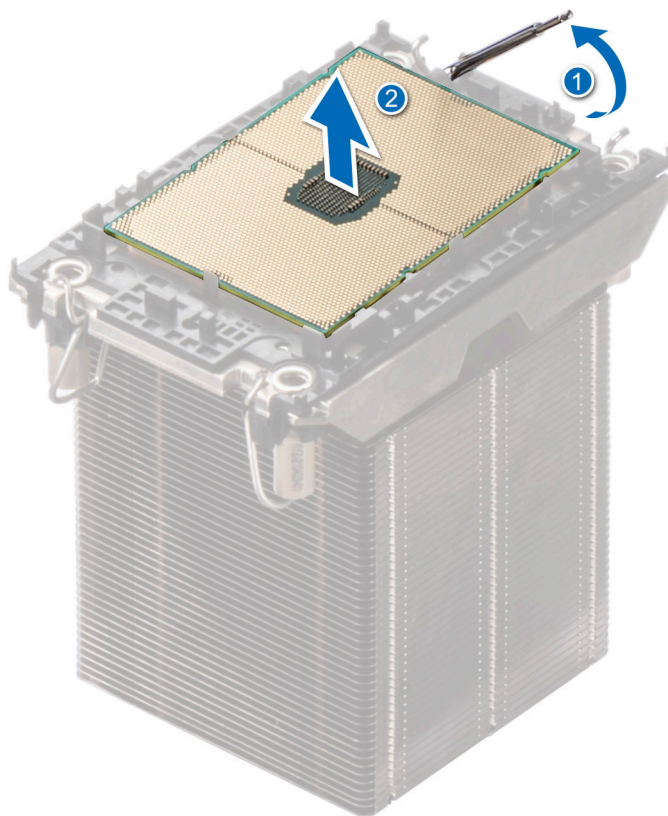
Ilustración 142. Levante la palanca de liberación del TIM
