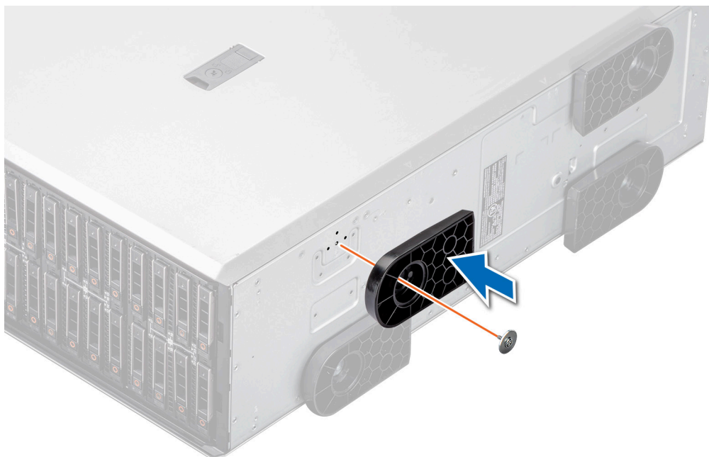
Ilustración 28. Instalación de los pies del sistema
