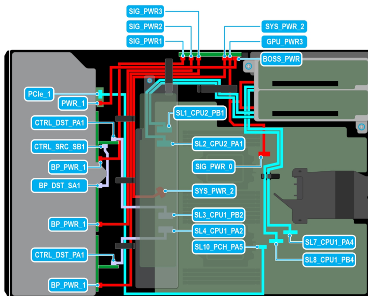
Ilustración 83. Enrutamiento de cables: 24 SAS de 2,5 pulgadas con dos soportes verticales para la GPU
