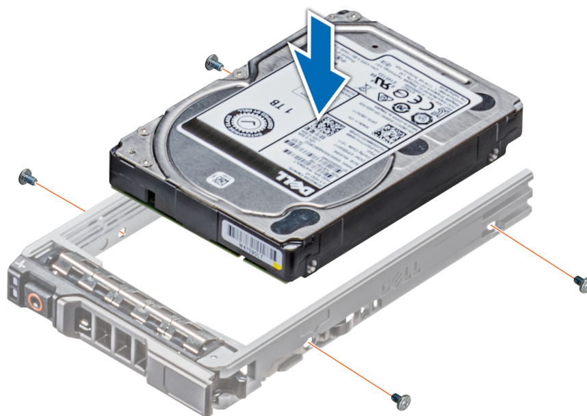
Ilustración 51. Instalación de una unidad en el portaunidades
