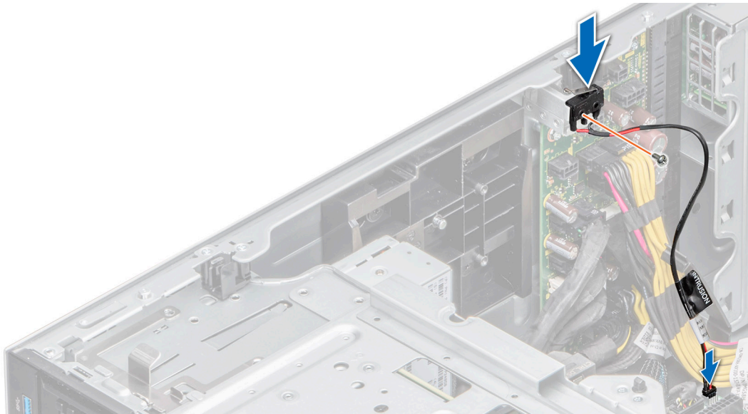
Ilustración 162. Instalación del módulo del interruptor de intrusiones
