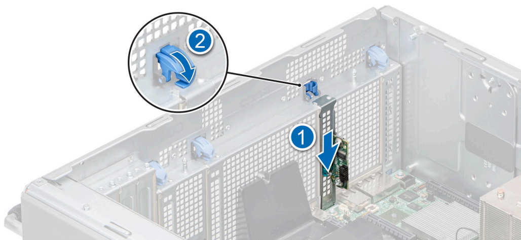
Ilustración 158. Instalación del puerto serie COM
