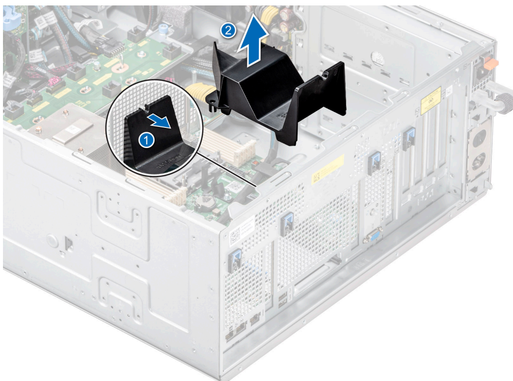
Ilustración 151. Extracción de la cubierta para flujo de aire de OCP
