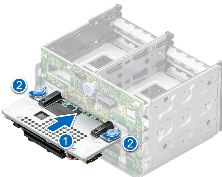
Ilustración 45. Instalación del módulo de PERC frontal en backplanes para unidades de 2,5 pulgadas.
