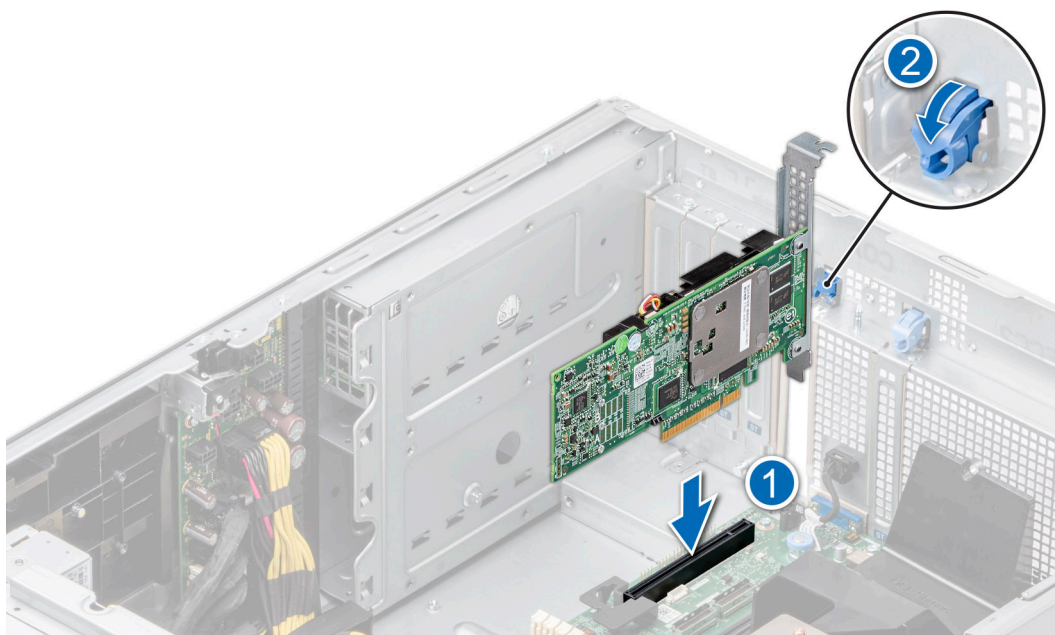
Ilustración 131. Instalación de una tarjeta de expansión
