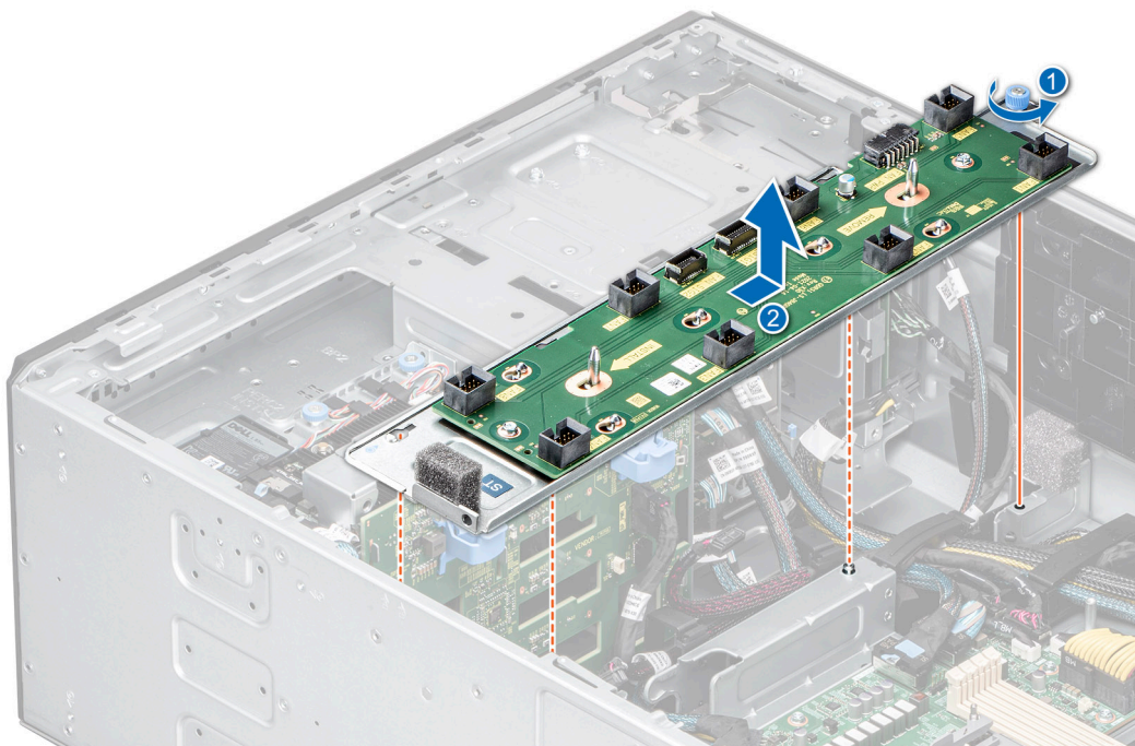
Ilustración 40. Extracción de la bandeja de la placa del ventilador
