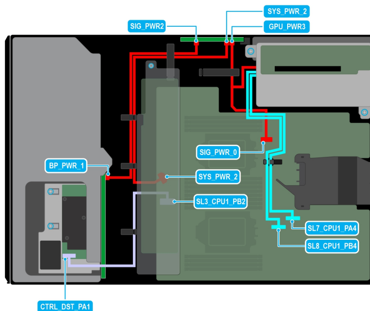
Ilustración 86. Enrutamiento de cables: 8 SAS de 3,5 pulgadas con soporte vertical para la GPU
