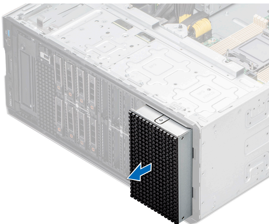
Ilustración 63. Extracción de la canastilla de relleno de la bahía de unidad
