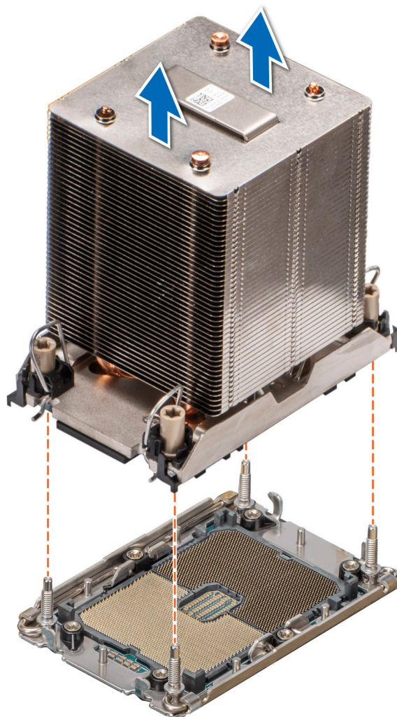
Ilustración 141. Extracción de un disipador de calor
