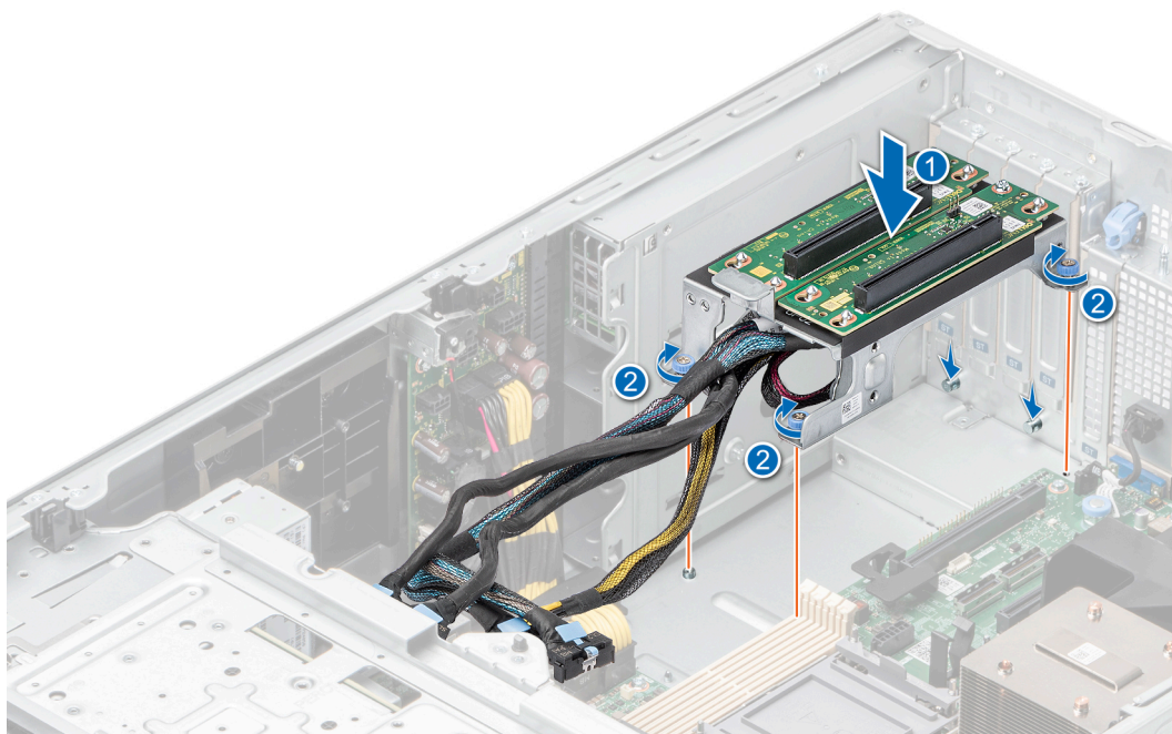
Ilustración 139. Instalación del soporte vertical de la GPU
