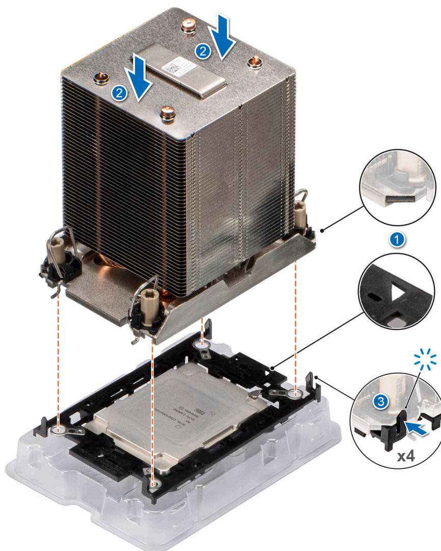
Ilustración 148. Instalación del disipador de calor en el procesador.
