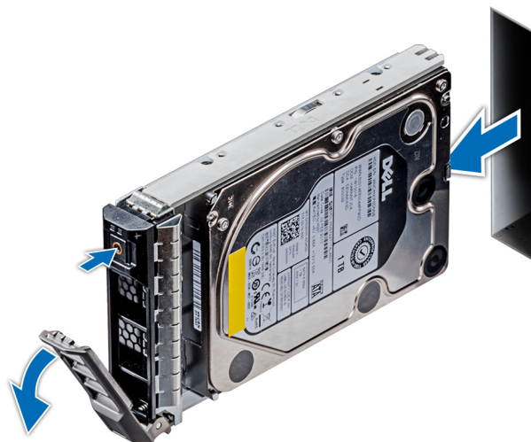
Ilustración 48. Extracción de un portaunidades
