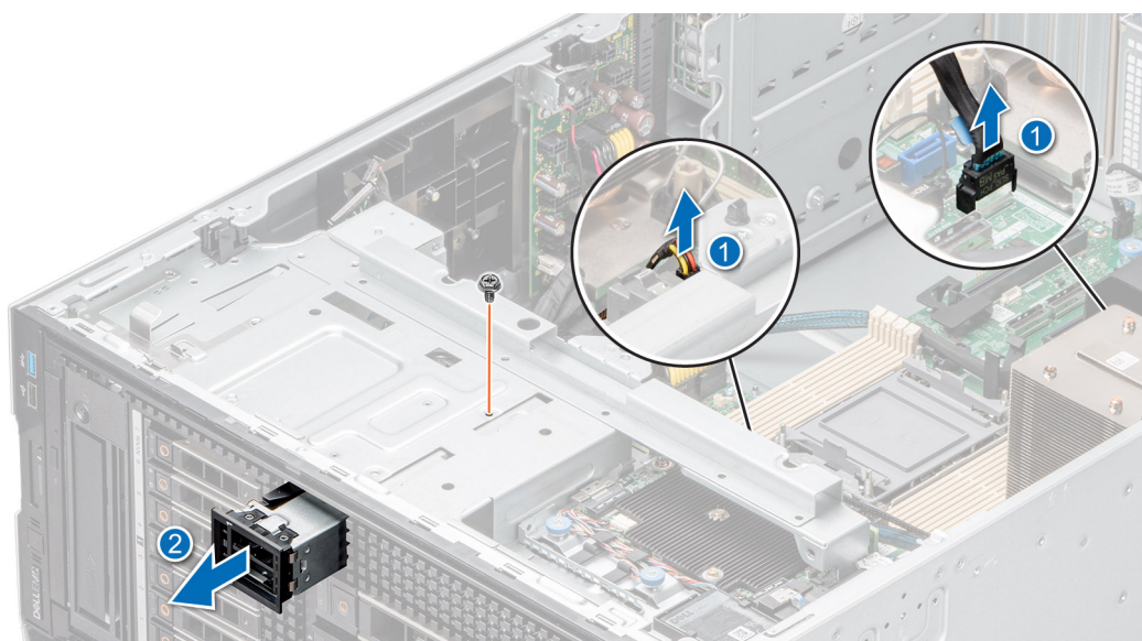
Ilustración 109. Extracción del módulo S2 de BOSS
