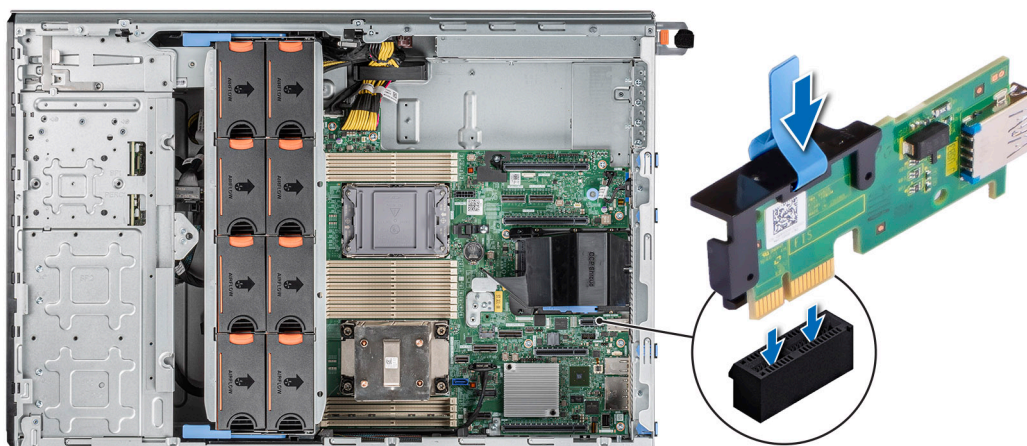
Ilustración 121. Instalación del módulo USB interno
