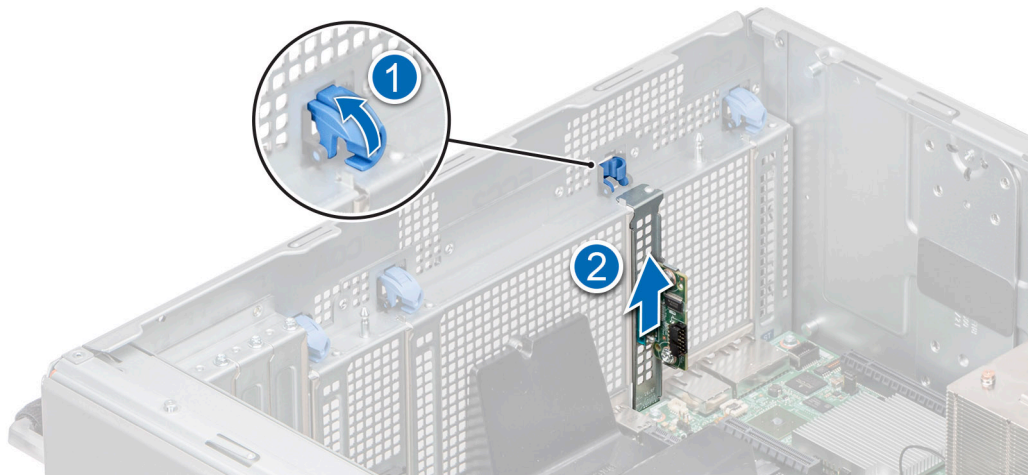
Ilustración 157. Extracción del puerto serial de COM
